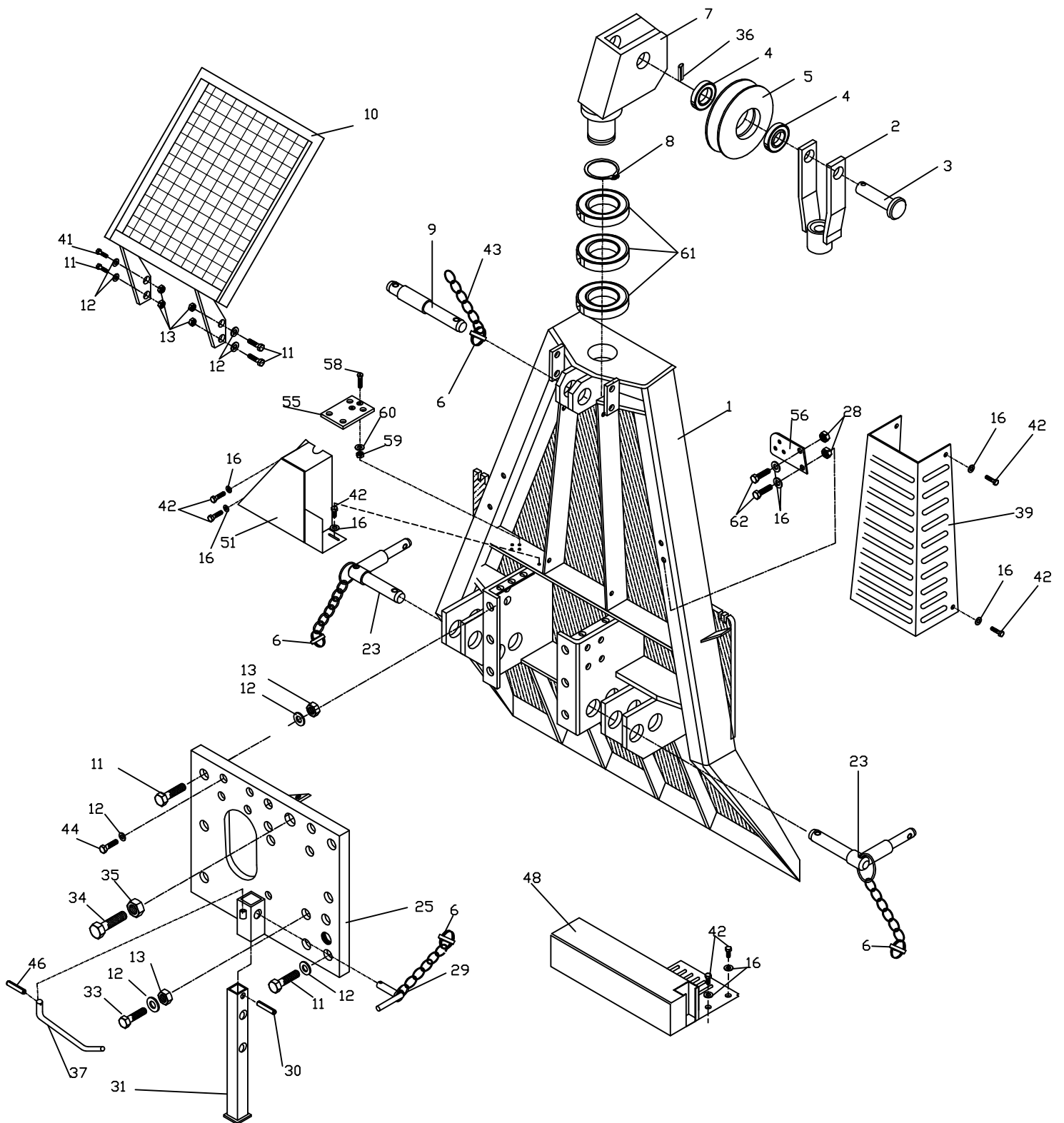
Ersatzteile Rückeschild HS-250 E
