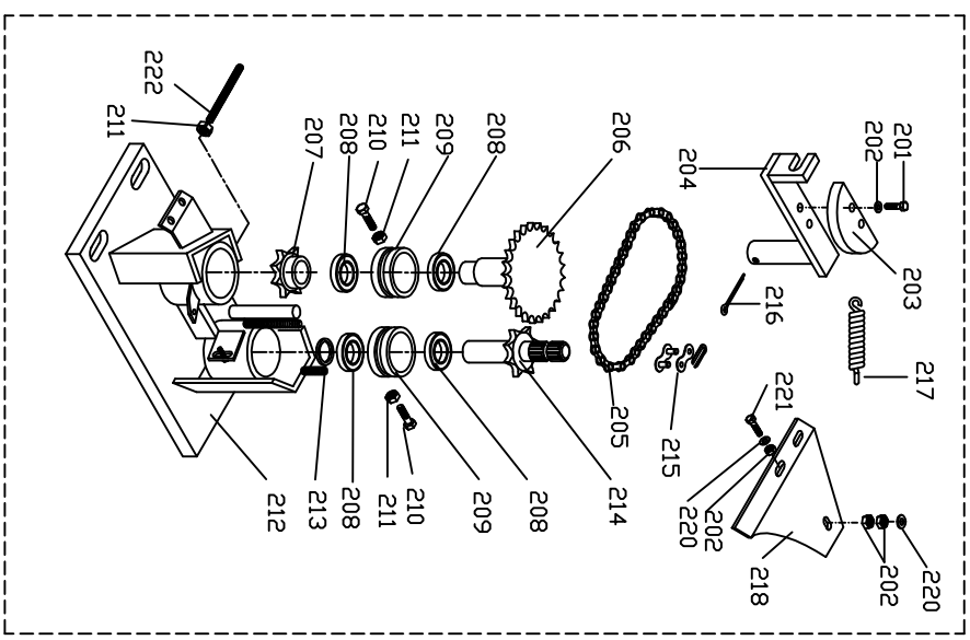
Ausführung - Unteretzungsgetriebe
